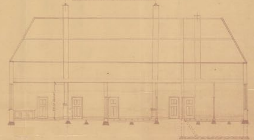
DOORSNEDEN A-B
