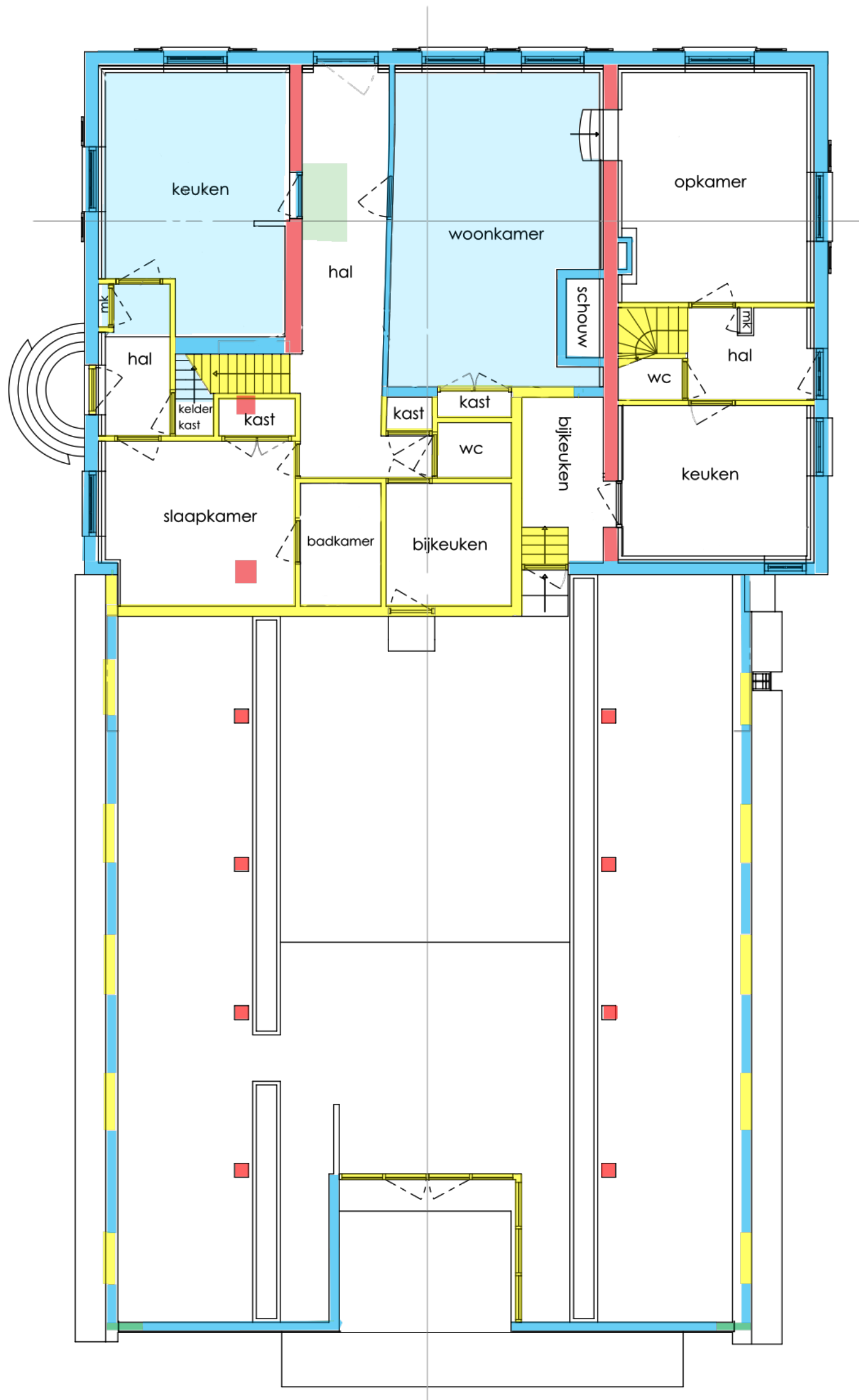
BEGANE GROND
