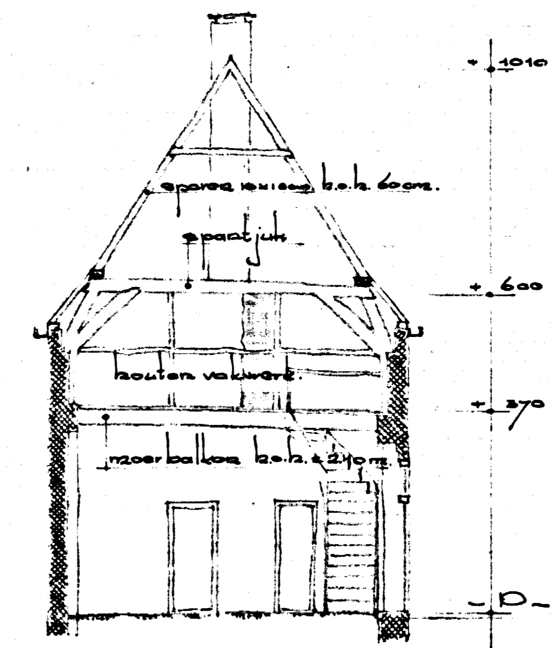
~ doorsnede a-b ~
