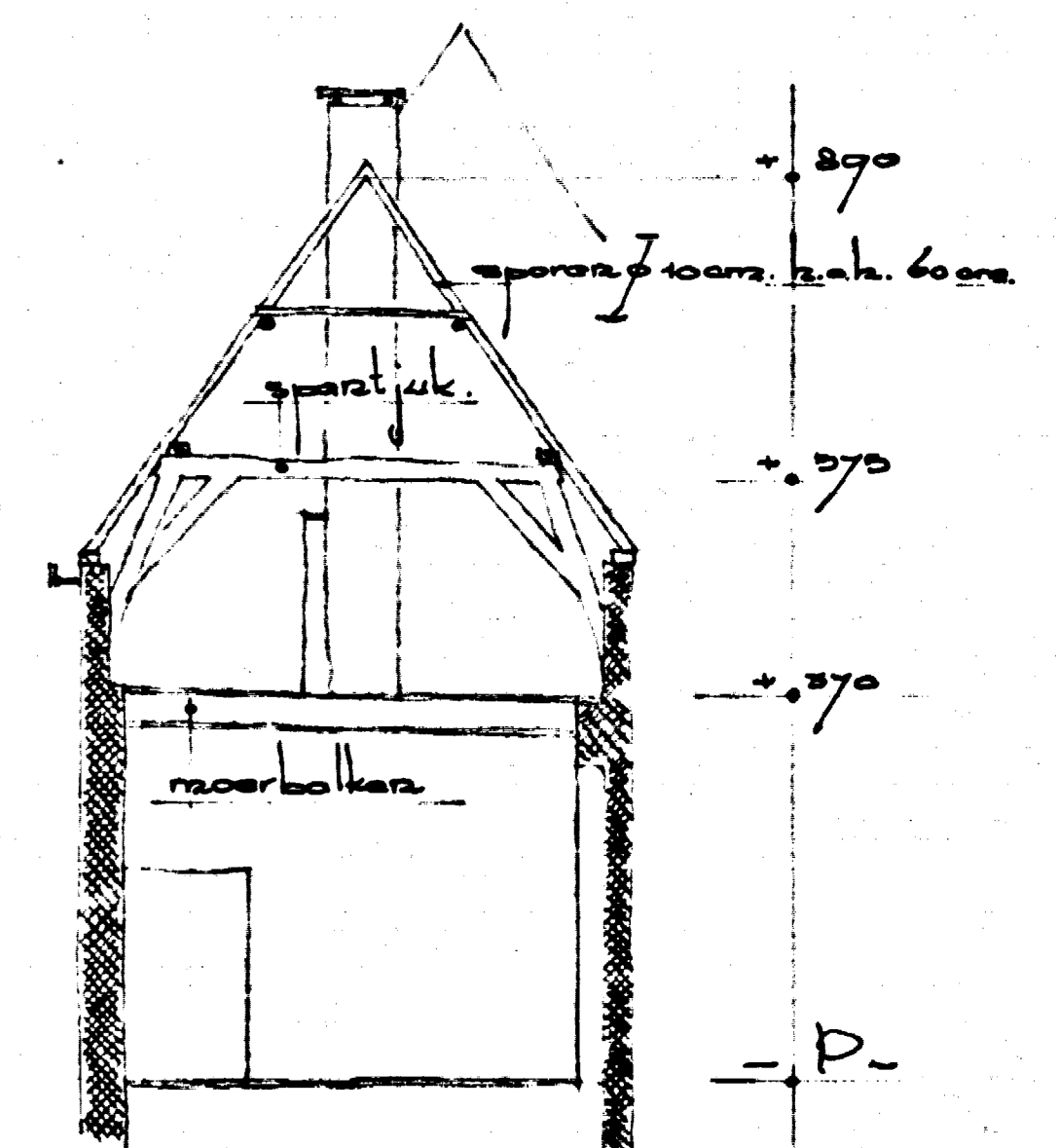
~ doorsnede c-d ~
