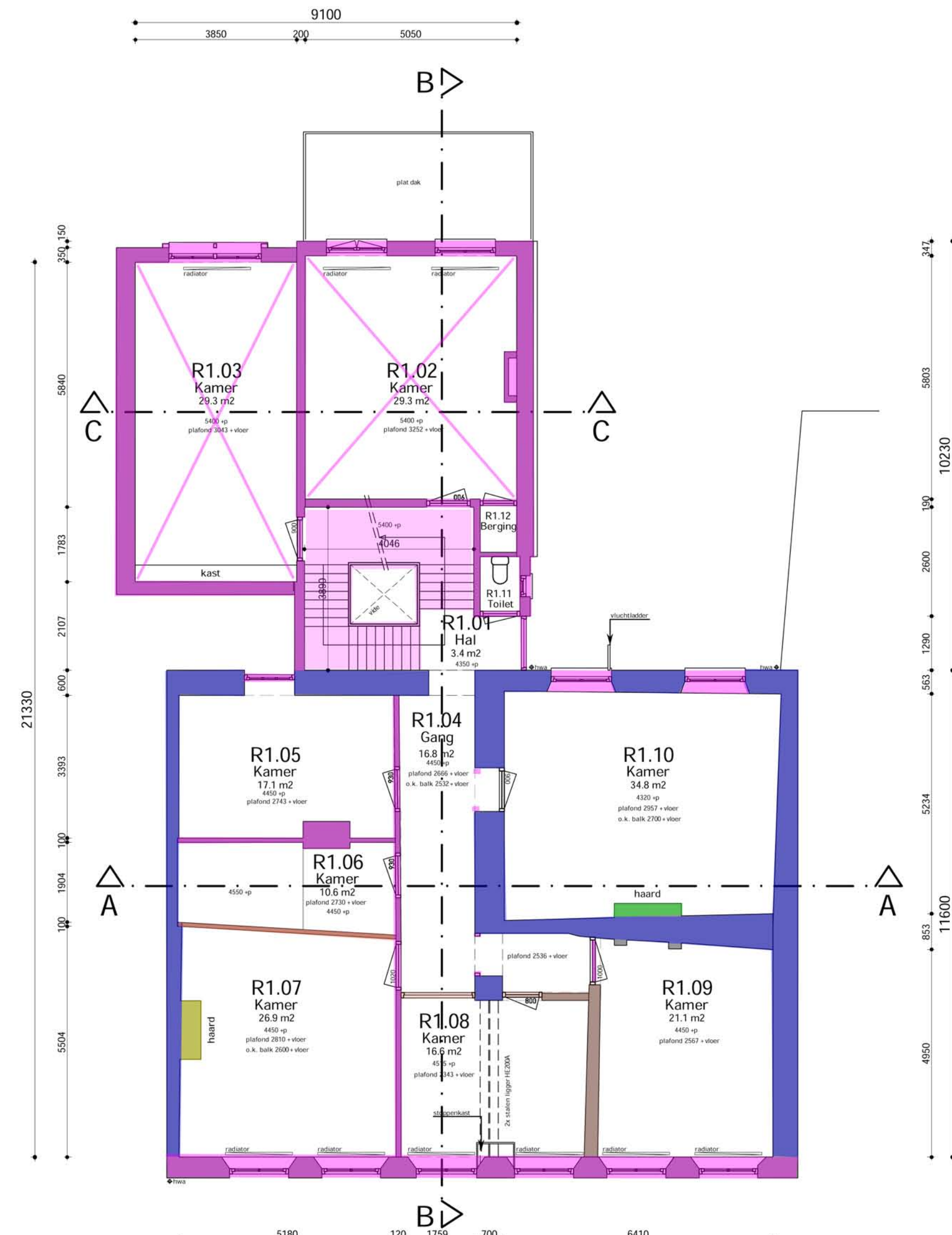
1e verdieping
