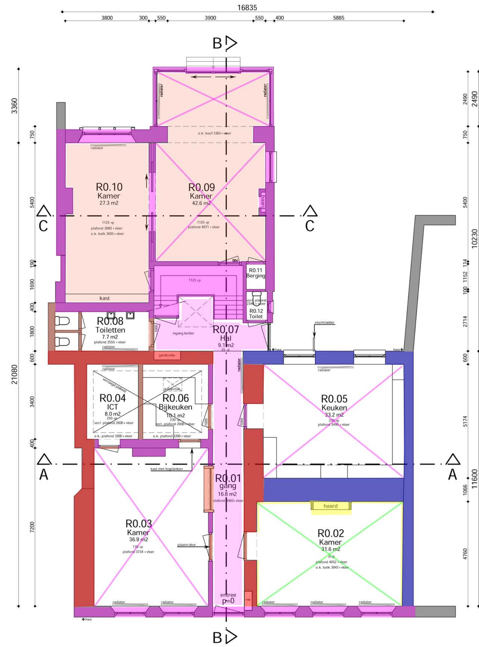
begane grond
