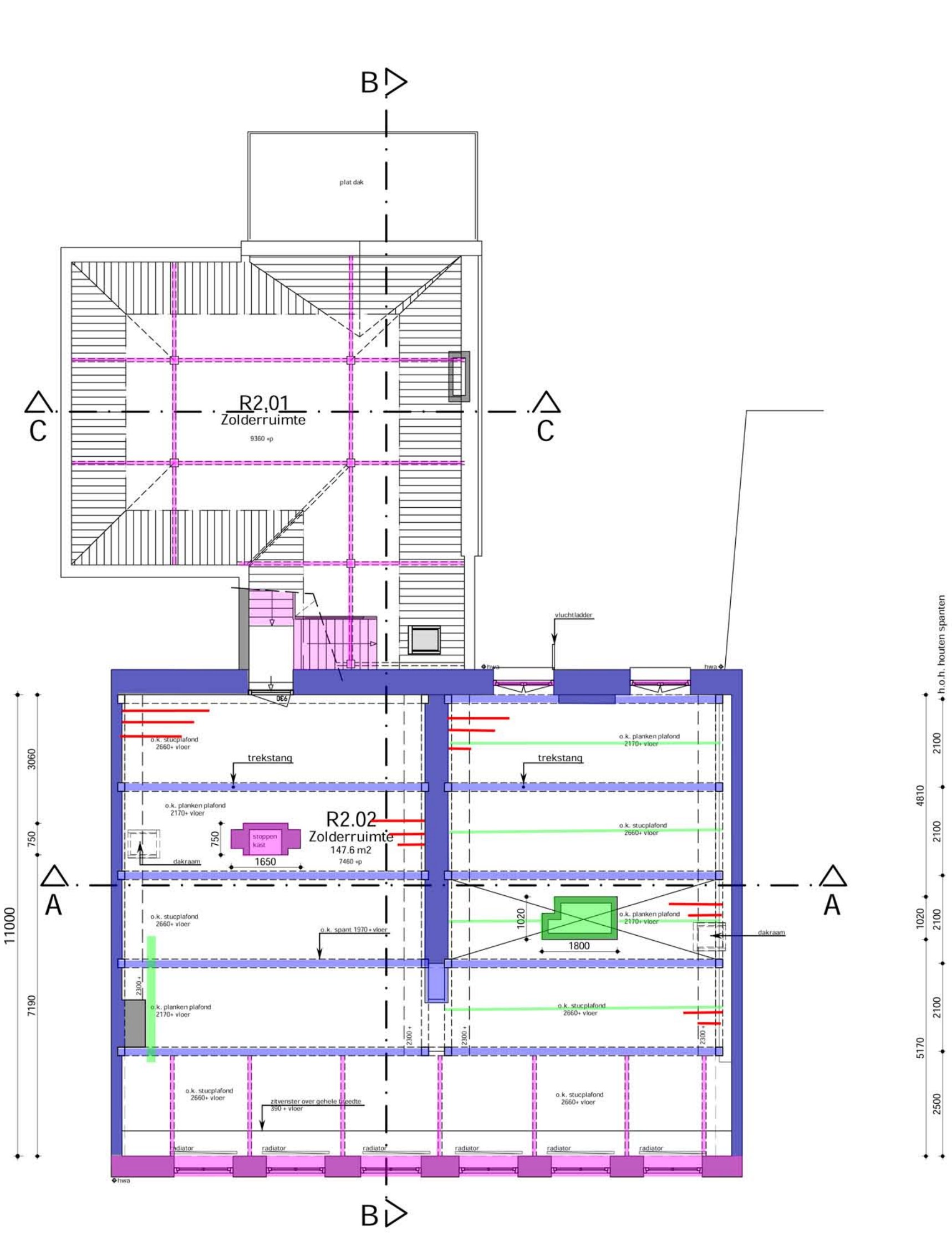
2e verdieping
