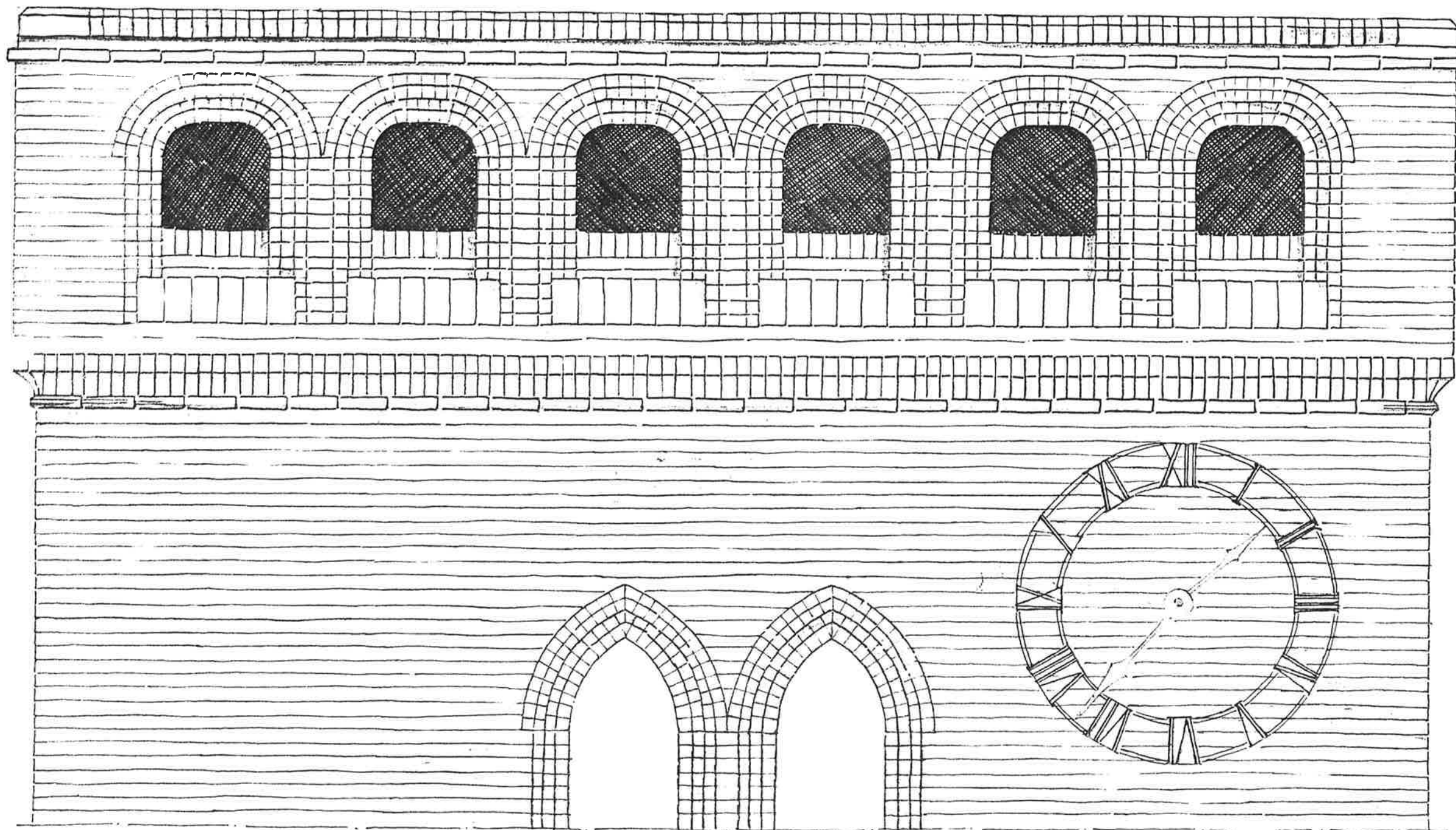
TORENTTRANS 1:20 na restauratie
