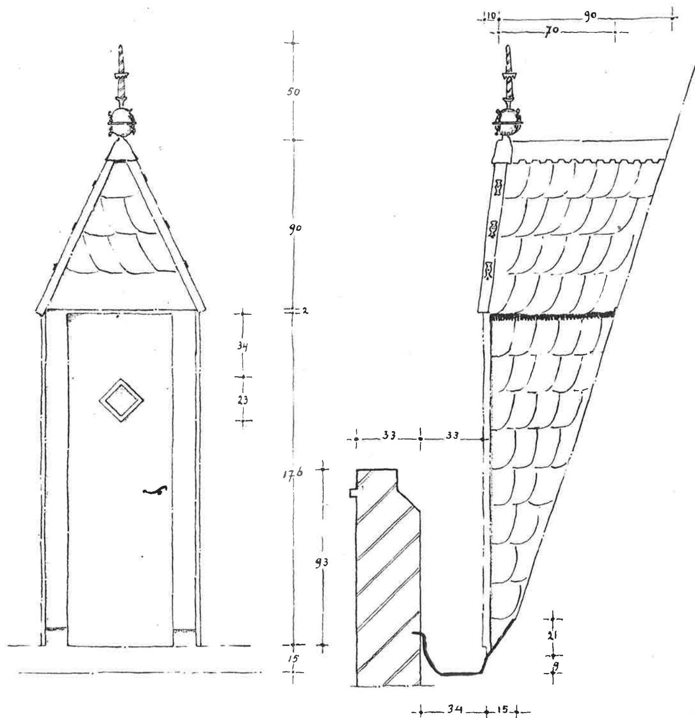
Dakkapel Torens spits 1:20
