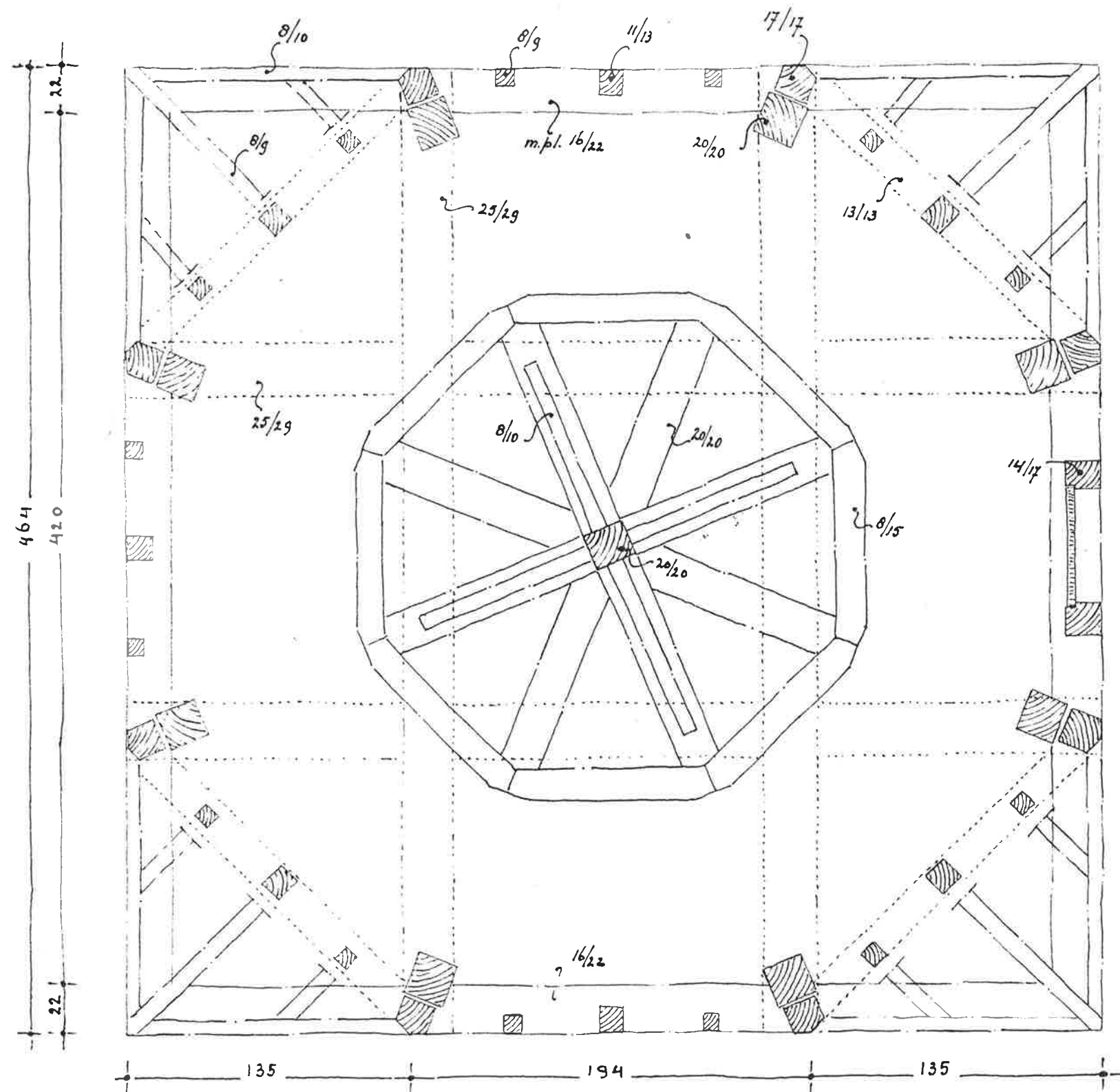
Plattegrond Torenspits 1:25
