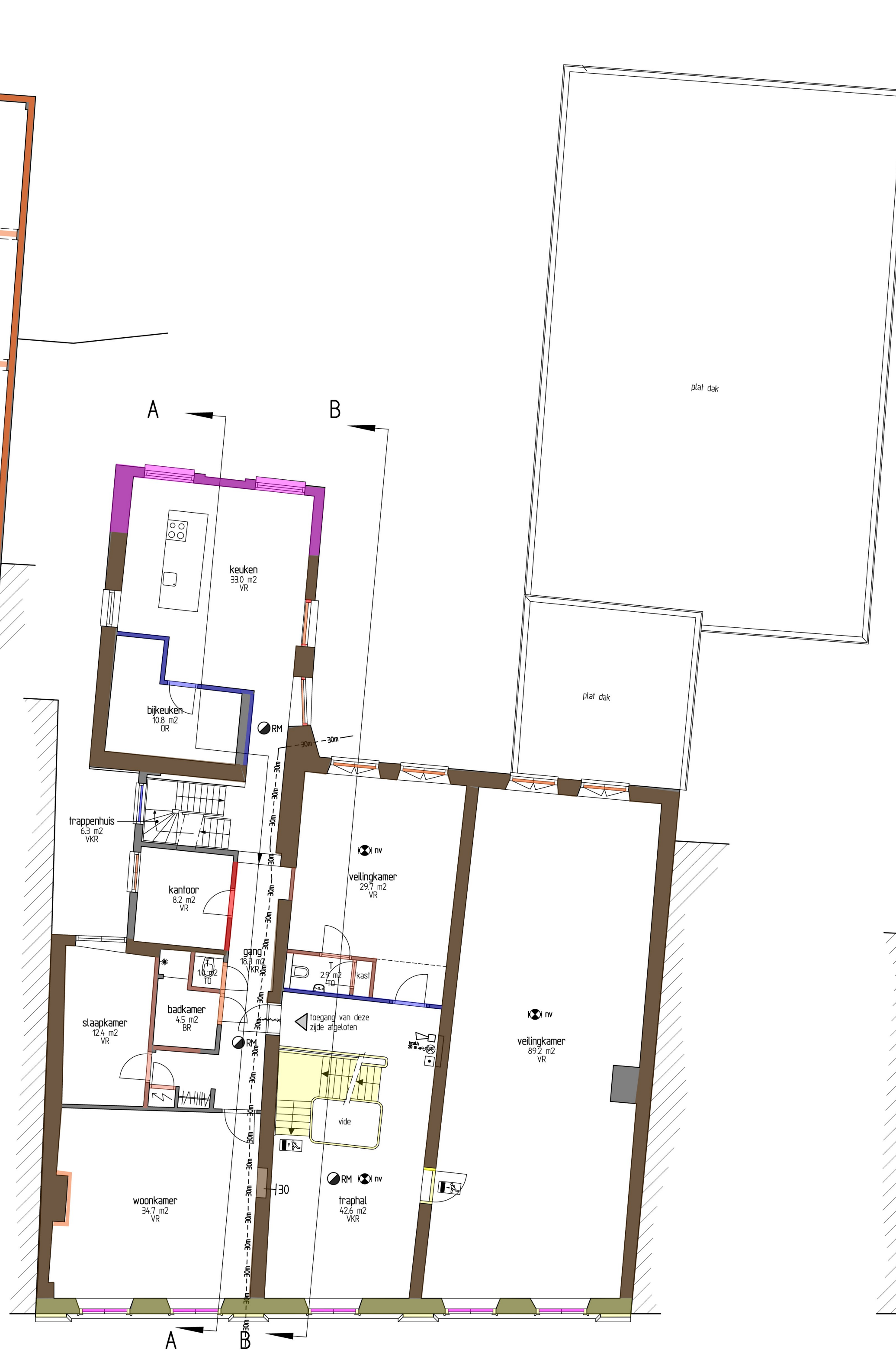
1e VERDIEPING B.V.O. ca. 355 m 2
