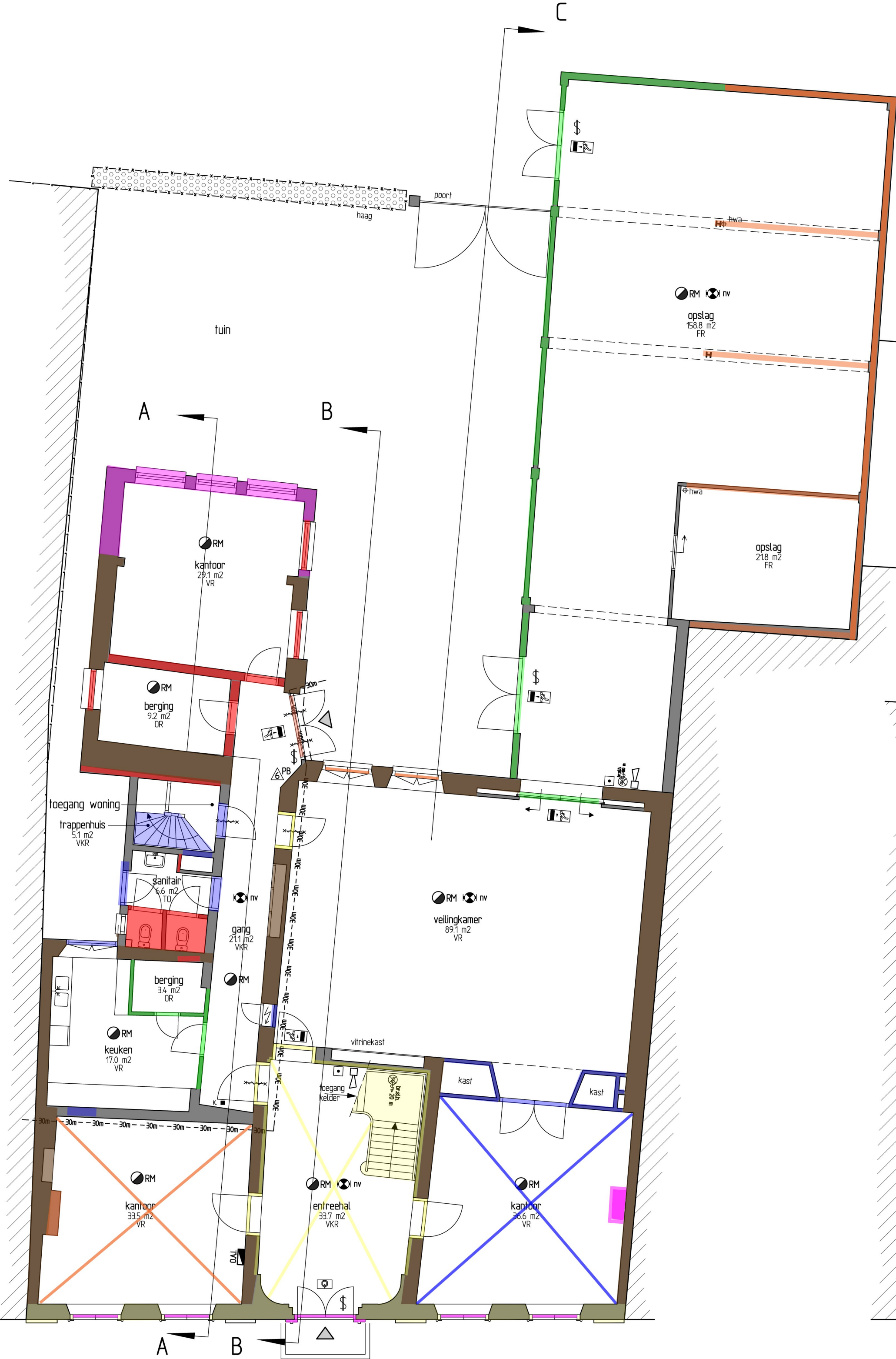
BEGANE GROND B.V.O. ca. 550 m 2
