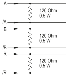
Abb. 8: Anschlusshinweis
