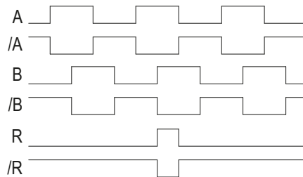
Abb. 9: Signalfolge
