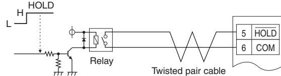
(d) Relay
