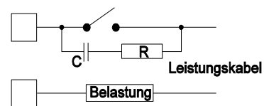
Abb.8 EXTERNER, ZUM AUSGANG DES GERÄTS IN REIHE GESCHALTETER KONTAKT
