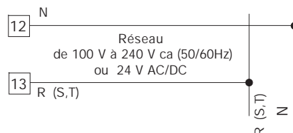
Fig. 10 RACCORDEMENT A L'ALIMENTATION
