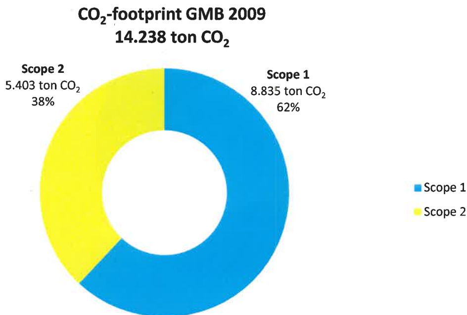
Afbeelding B-III.1: directe en indirecte CO 2 emissies (scope 1 en 2)
