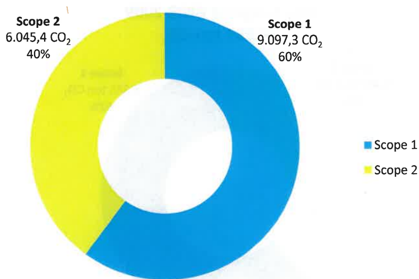
Afbeelding B-III.2: directe en indirecte CO 2 emissies 2009 herberekend (scope 1 en 2)
