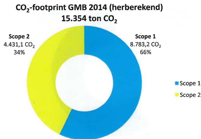
Afbeelding B-IV.2: directe en indirecte CO 2 emissies 2014 herberekend (scope 1 en 2)
