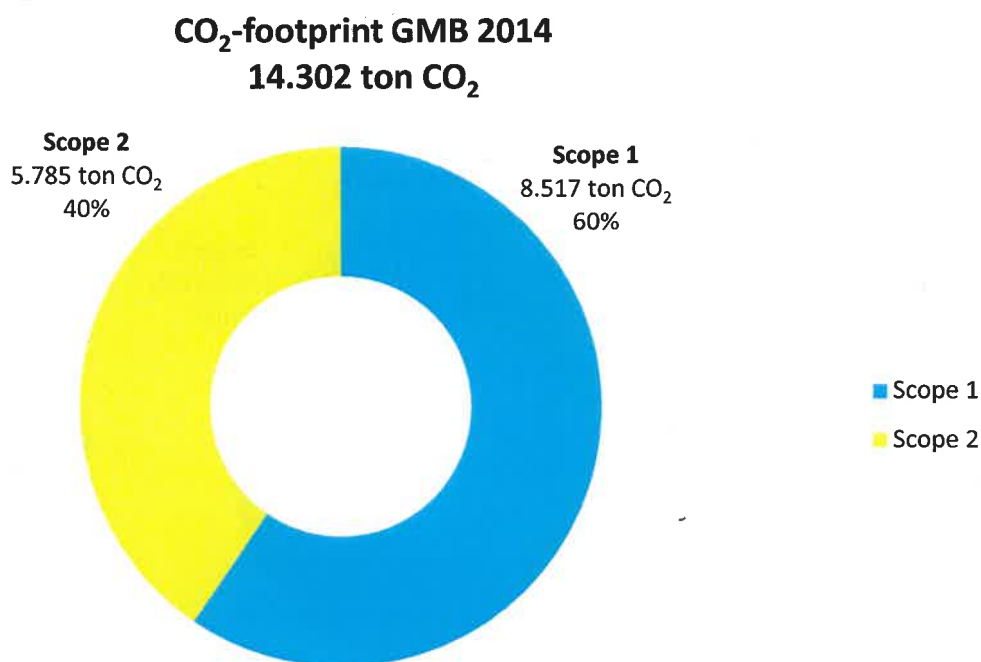
Afbeelding B-IV.1: directe en indirecte CO 2 emissies 2014 (scope 1 en 2)
